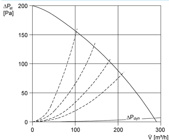
ERM 18 E Ex Ydelses graf
