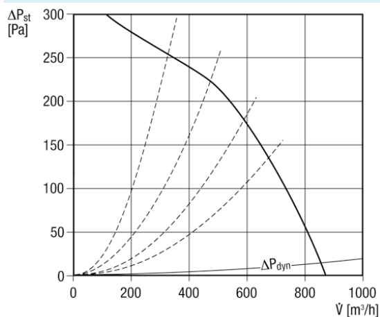
ERM 25 E Ex Ydelses graf
